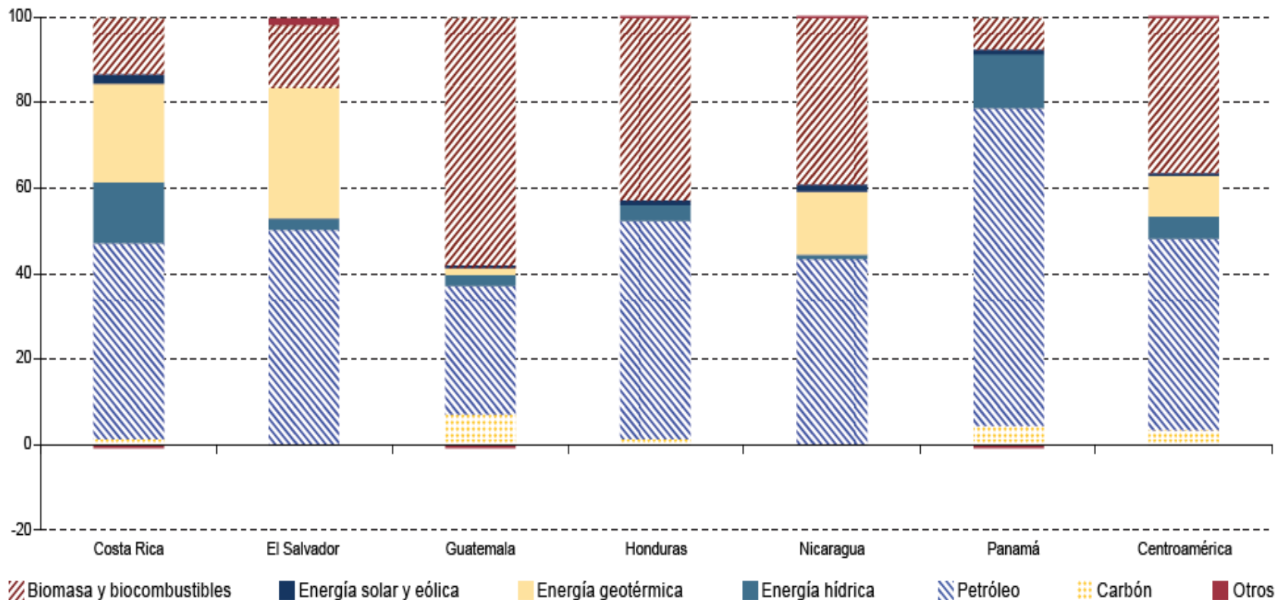
Centroamérica (6 países): composición de la matriz energética por país, 2015 (En porcentajes)
