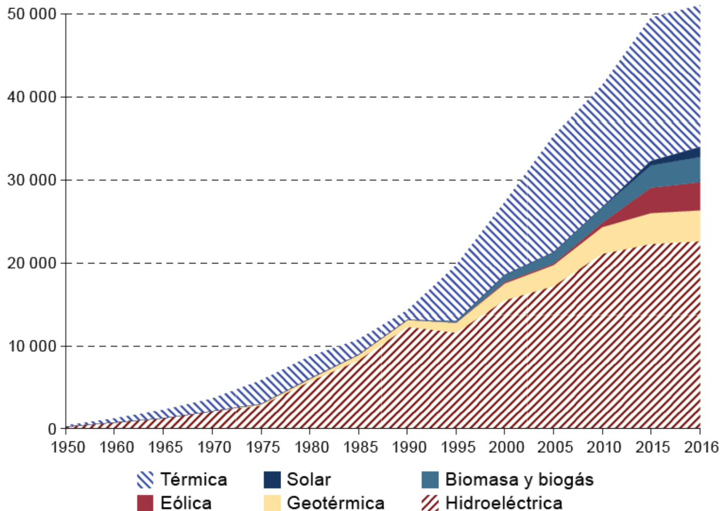
Centroamérica: producción de energía eléctrica, por fuentes, 1950-2016 (En gigavatios por hora)
