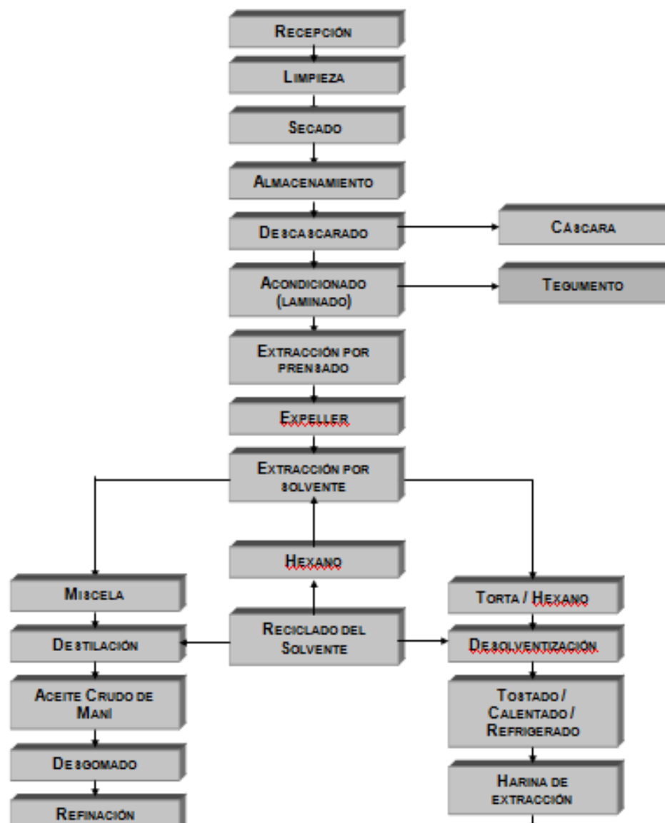
DIAGRAMA DE PROCESO
