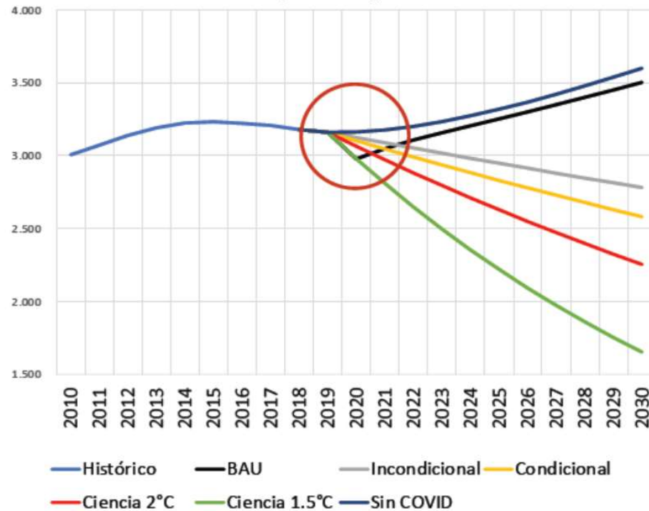
América Latina y el Caribe: Emisiones 2030 bajo distintos escenarios, 2010-2030 (MtCO 2 eq)
